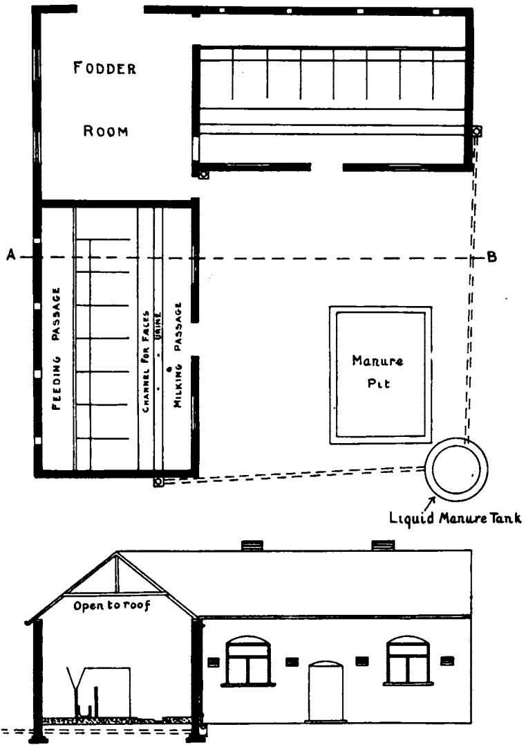
Section A.B.
