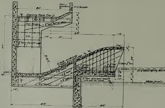
Fig. 6 Municipal Natatorium, San Jose. H. J. Brunner, C. E.
