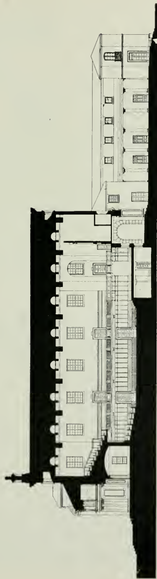
LONGITUDINAL SECTION
