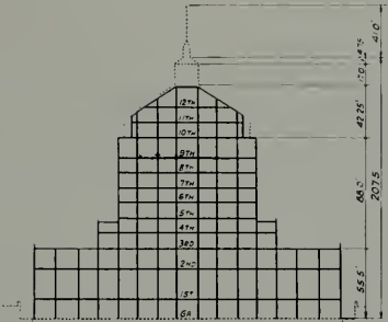
LONGITUDINAL SECTION STEEL
