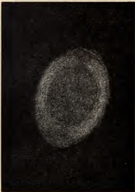
Fig. 80.—The Ring Nebula.
