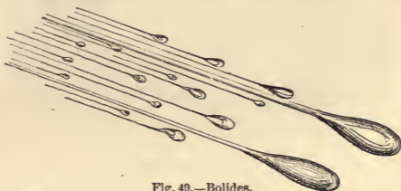
Fig. 49.—Bolides.
