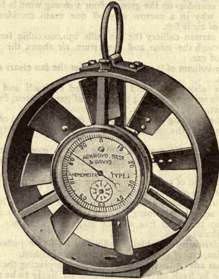
FIG. 38.—Anemometer.
