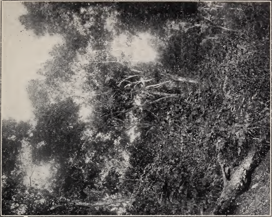
Fig. 2.—Guamá. Inga laurina .
