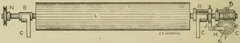
Fig. 88. Long Roll Grinder.
