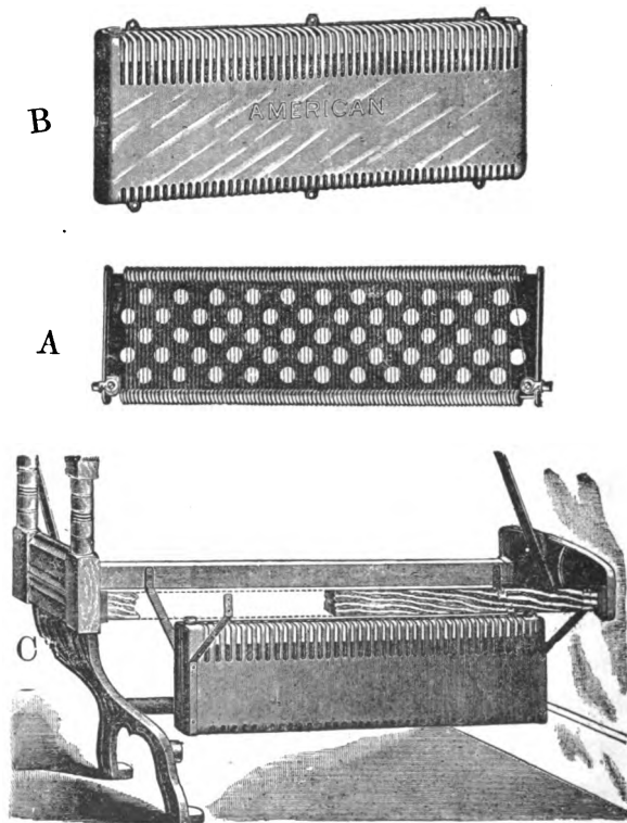
FIG. 29.—CAR-HEATER.
