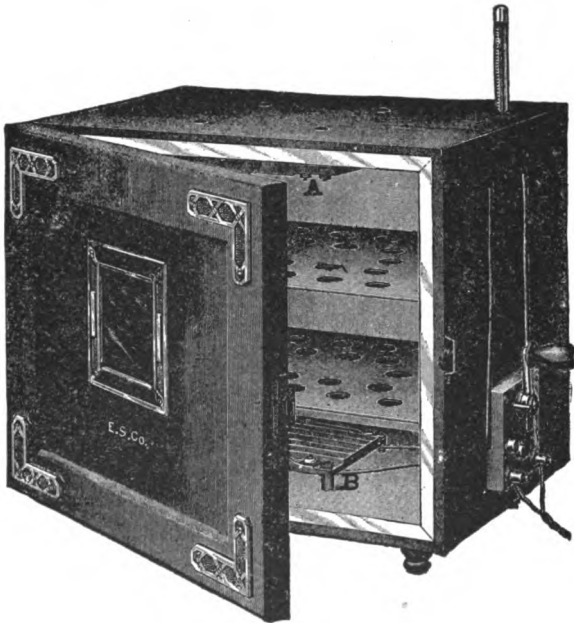
FIG. 41.—ELECTRIC OVEN.
