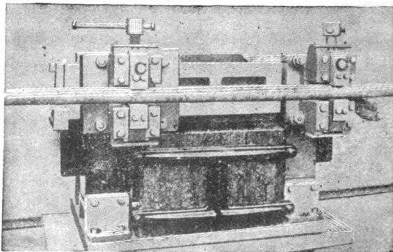
FIG. 73.—PIPE-BENDING APPARATUS.
