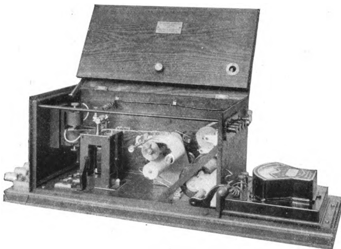
Fig. 25a. — G. E. RECORDING AMMETER.
