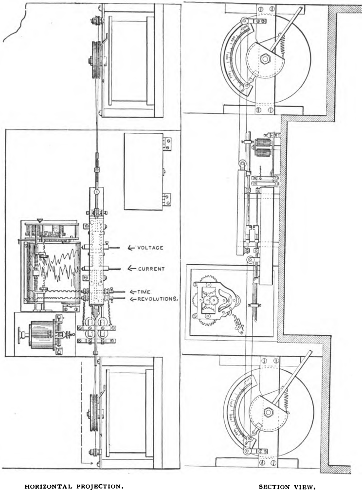
Fig. 20. — KEILEY RECORDER.
