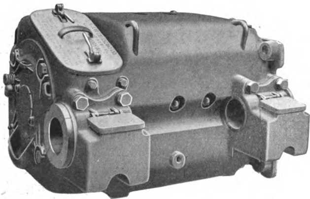
Fig. 45. — G. E. 66 RAILWAY MOTOR.
