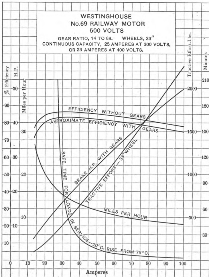
Fig. 37. — MOTOR CURVE.
