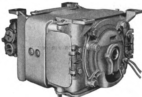
Fig. 152. — G. E. MOTOR DRIVEN AIR COMPRESSOR.
