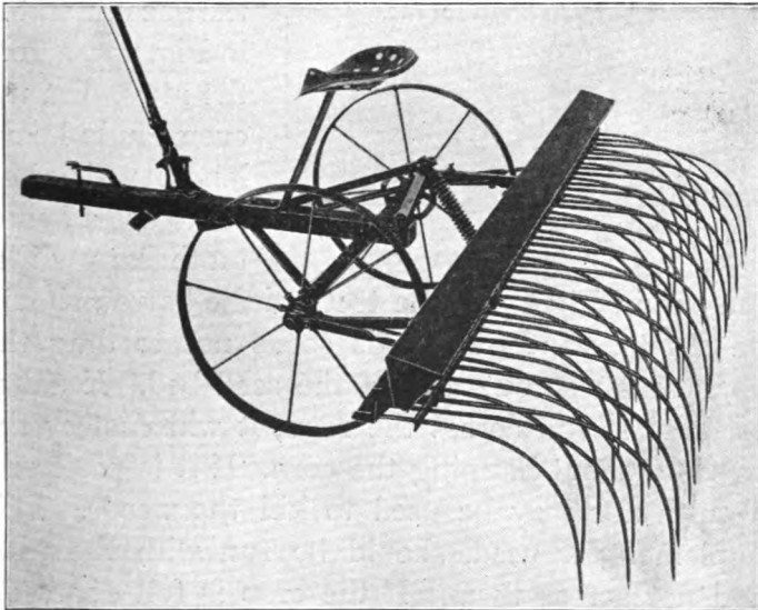
FIG. 157. A WEEDER
