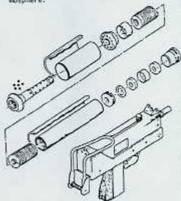
SUPPRESSOR M11 3MM PARA. C 45ACP
