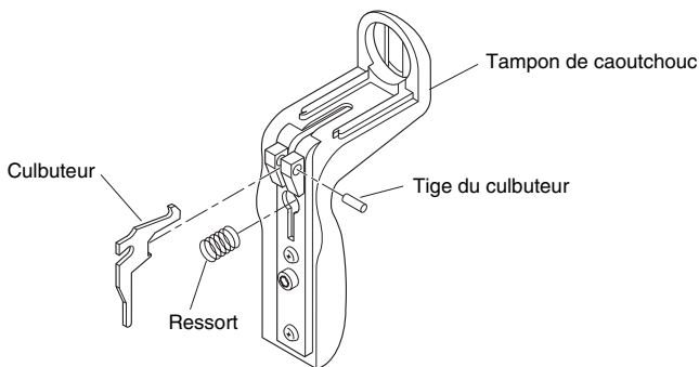
Figure 6 - Retrait du culbuteur
