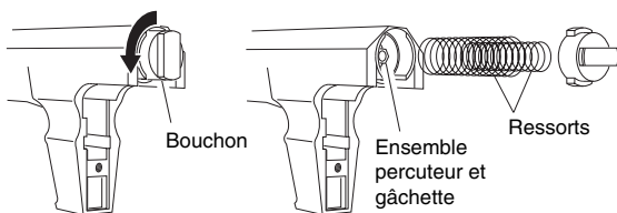
Figure 7 - Retrait du bouchon et des ressorts pour accéder au percuteur
