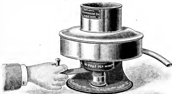
FIG. 2. De Laval's butyrometer.
