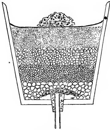
Fig. 80.—Filter.
