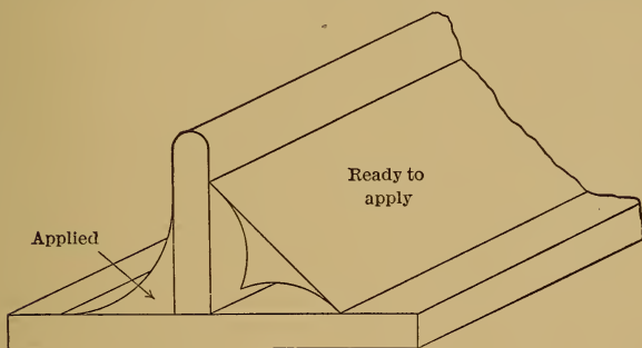
FIG. 41.—Leather Fillet.
