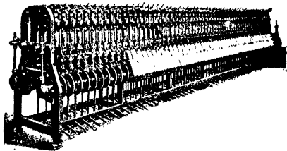
Cop Winding Machine Cops-Spinnmaschine Pinnmaschinenbau Hannover
