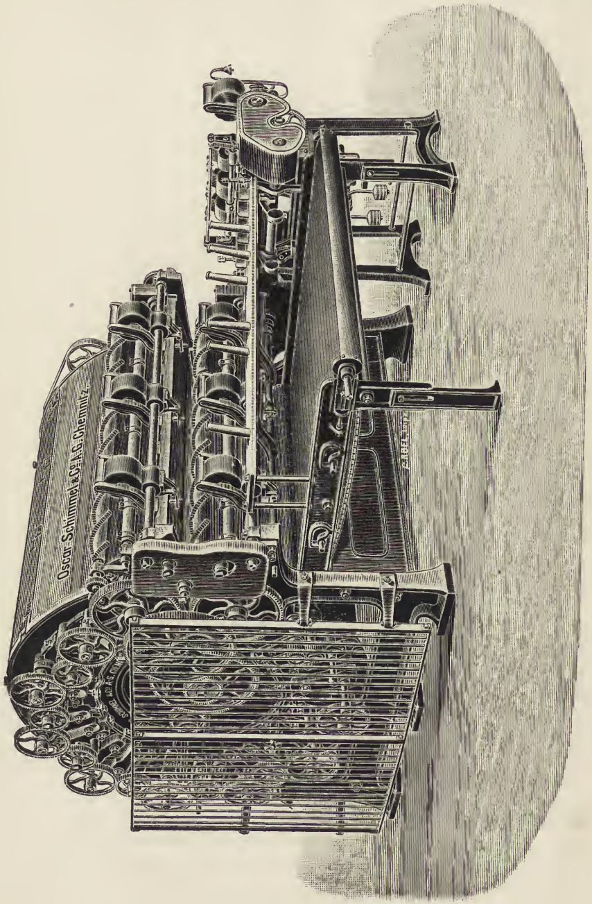
FIG. 33.—Tow card.
