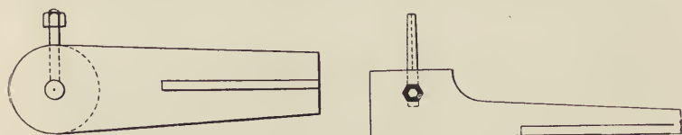
FIG. 9.—Touch pin.
