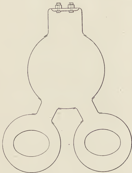
FIG. 150.—Section through a French generateur à bouilleurs.
