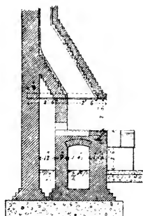
Longitudinal Section
