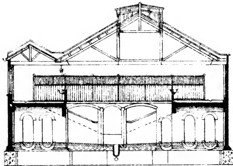
SECTION A. B.
