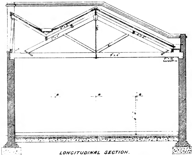
LONGITUDINAL SECTION.
