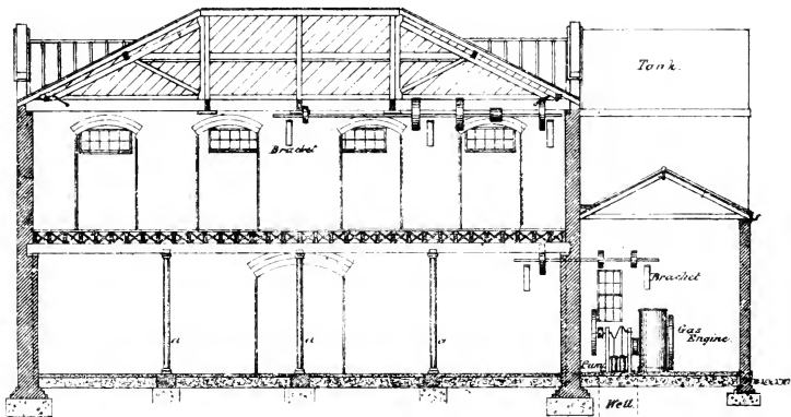
LONGITUDINAL SECTION THRO' CORN STORE.
