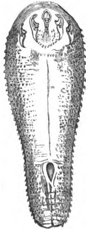
Fig. 24. LARVAL PENTASTOME.
