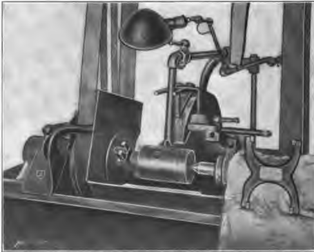
Fig. 29. Grinding Pistons
