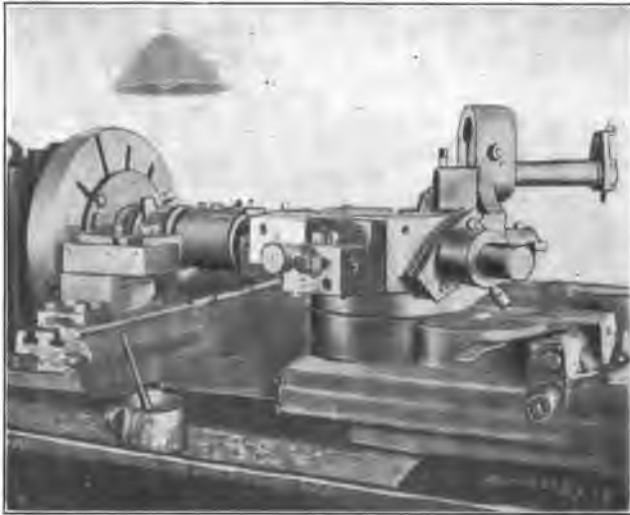
Fig. 26. Turning Cylinders
