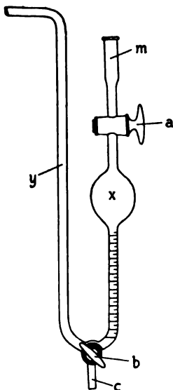
FIG. 112.—FRIDERICIA APPARATUS.
