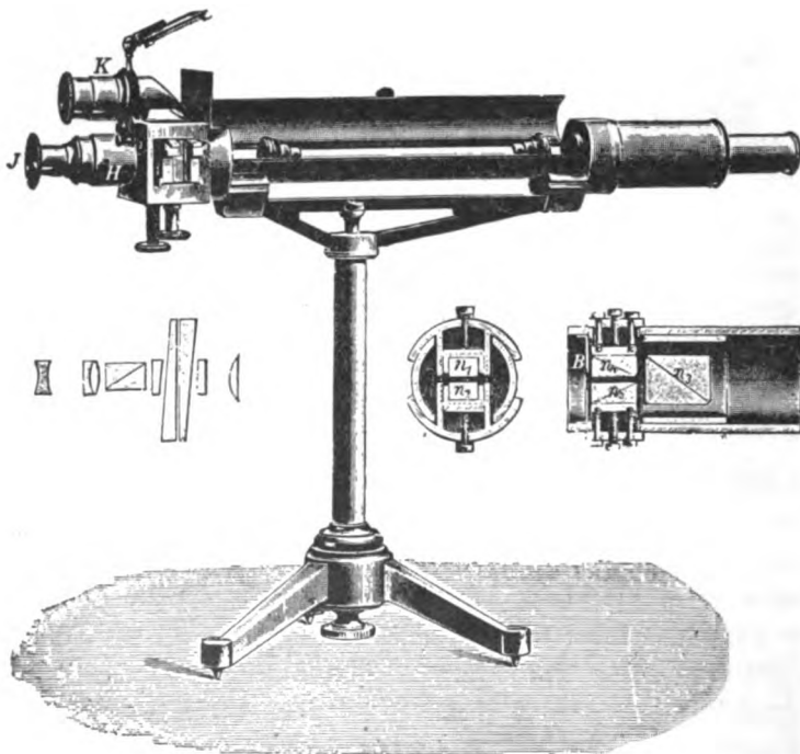
FIG. 8.—POLARISCOPE (SCHMIDT AND HÄNSCH MODEL).
