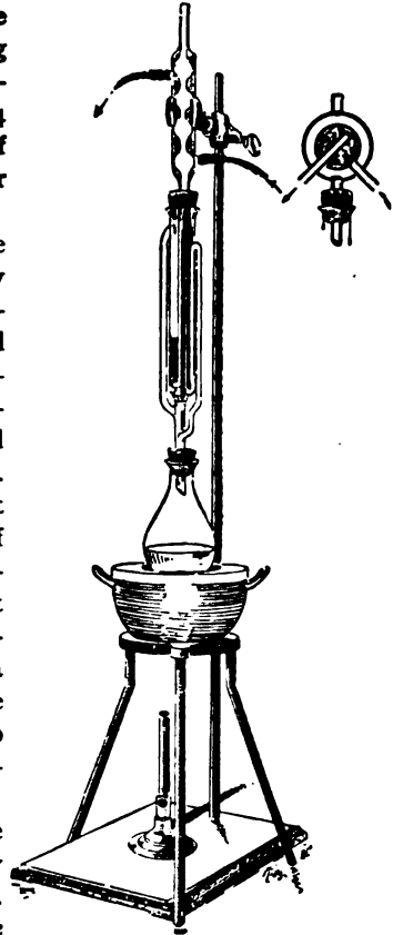
FIG. 122.—SOXHLET APPARATUS.
