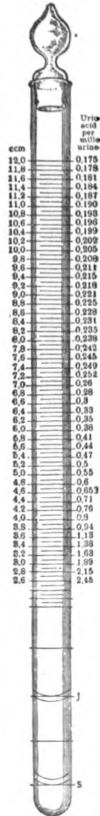
FIG. 176.—RUHEMANN'S URICOMETER.
