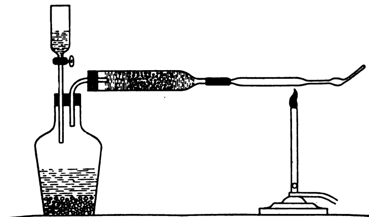
FIG. 146.—MARSH APPARATUS.
