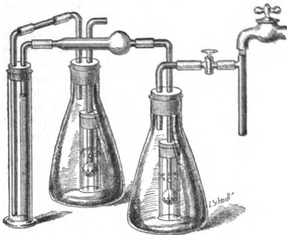
FIG. 174.—FOLIN AMMONIA APPARATUS.
