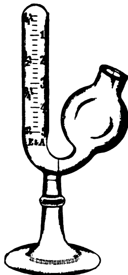
FIG. 5.—EINHORN SACCHAROMETER.
