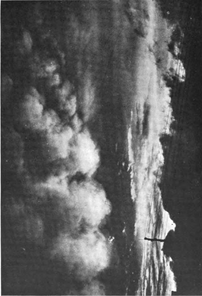
Atlas Photographique des nuages, Loisel.
