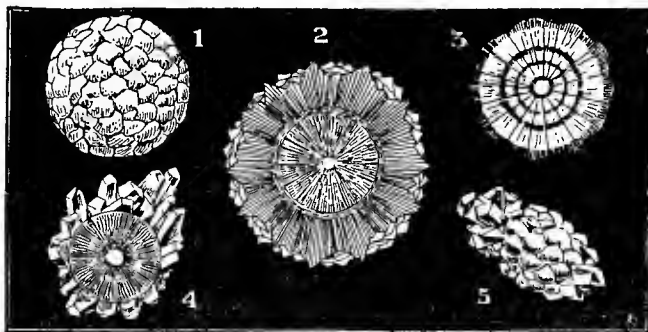
Fig. 68.—Hailstones
