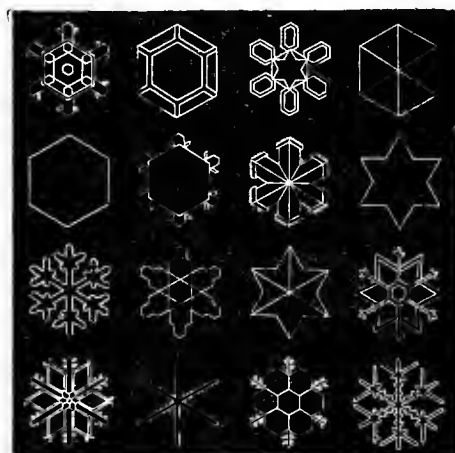
Fig. 67. — Snow Crystals
