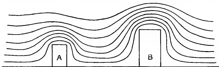
Fig. 87.—The Distortion of Equipotential Surfaces
