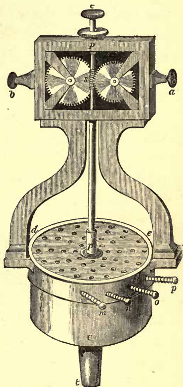
DOVE'S SIRENE.
