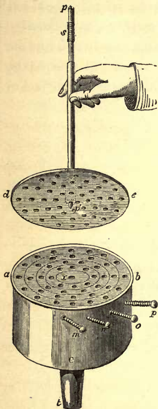
DOVE'S SIRENE.
