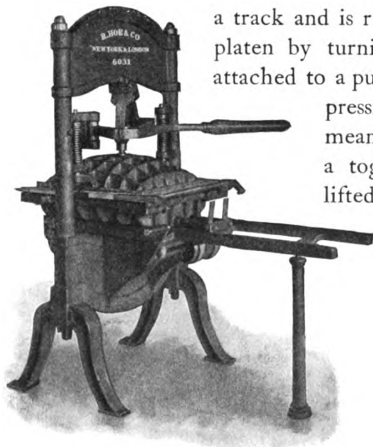
WASHINGTON HAND PRESS
