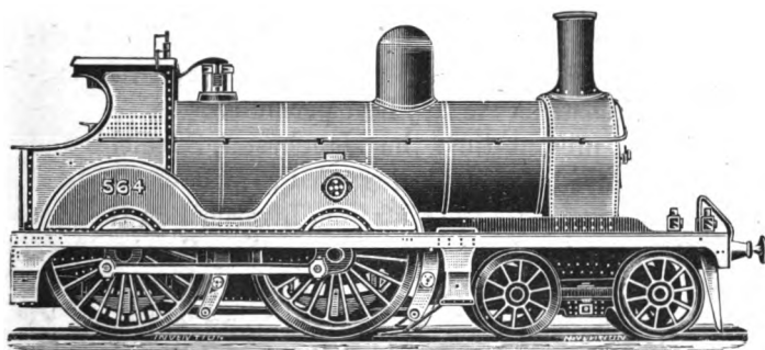
Fig. 80.—The Latest Design of M. S. & L. Express Engine.
