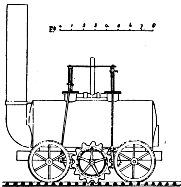
Fig. 2.—"Blenkinsop," 1812.
