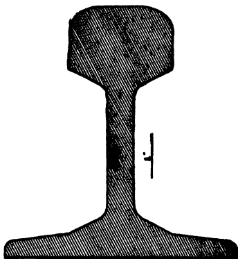
Stevens Rail, Chemin de fer du Nord. France, A. D. 1838.
