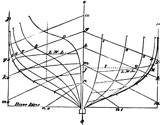
BODY PLAN.
