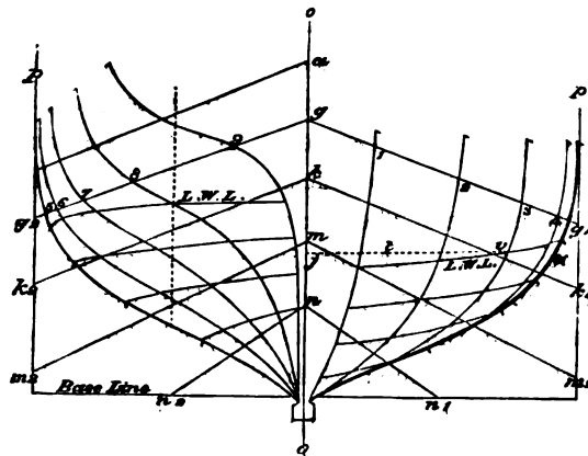
BODY PLAN.
