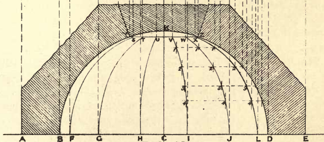
FIG. 12 — PLAN —
