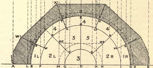
FIG. 7 PLAN
