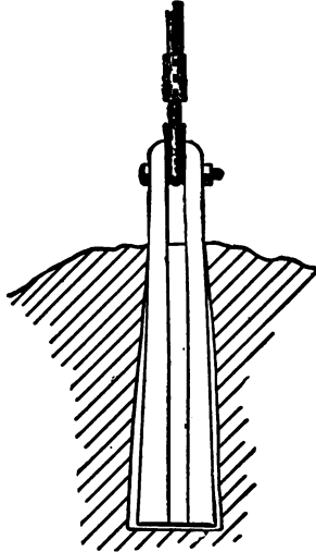
FIG. 101.— ROCK EYE-BOLT.
