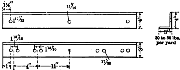
FIG. 56.— CABLE CROSS ARM.
