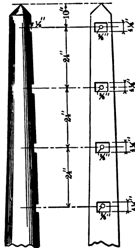
FIG. 50.— POLE TOP.
