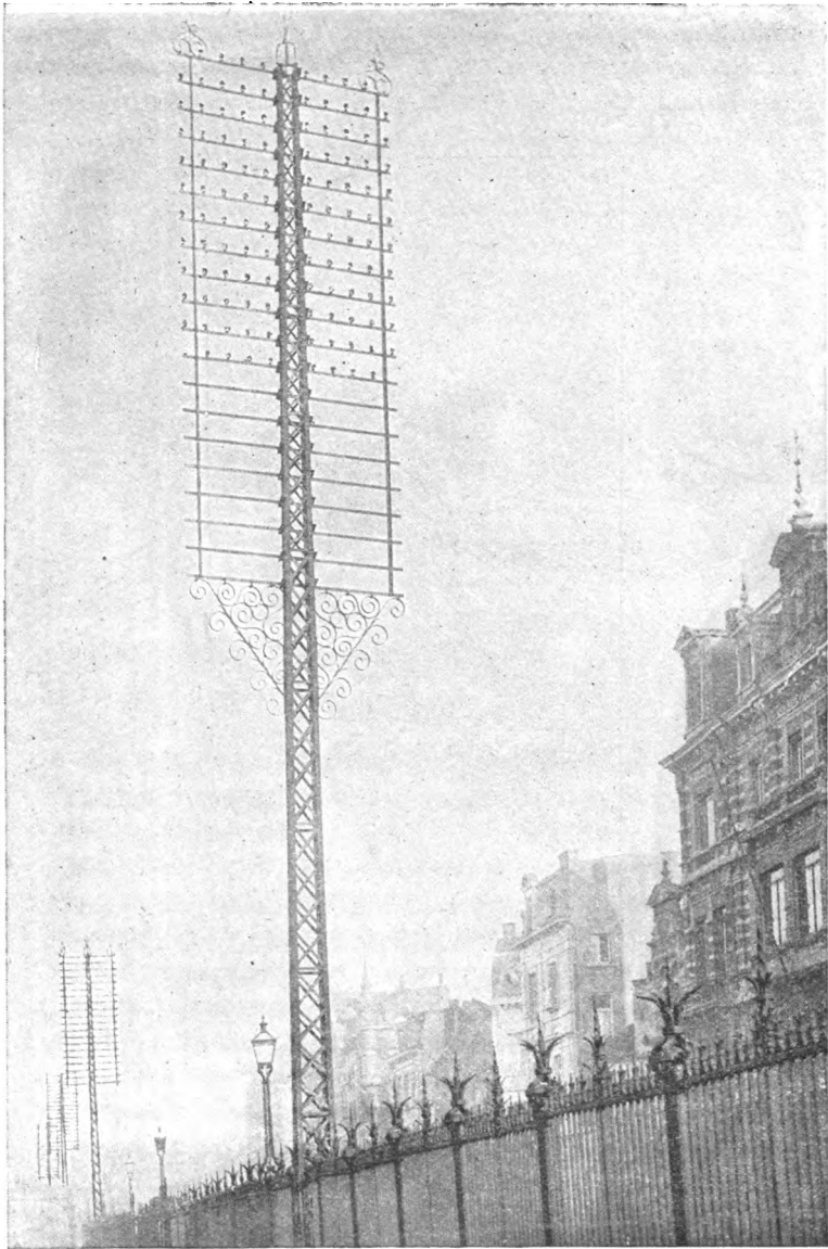
FIG. 13.— BELGIAN POLE LINE.
