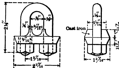
FIG. 57.— CABLE STRAND U-BOLT.
