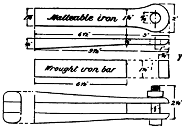
FIG. 78.— ROCK EYE-BOLT.
