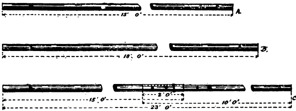
FIG. 134.— FIXTURE POLES.
