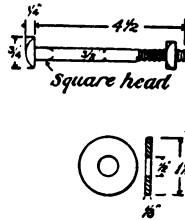
FIG. 66.—CARRIAGE BOLT.
