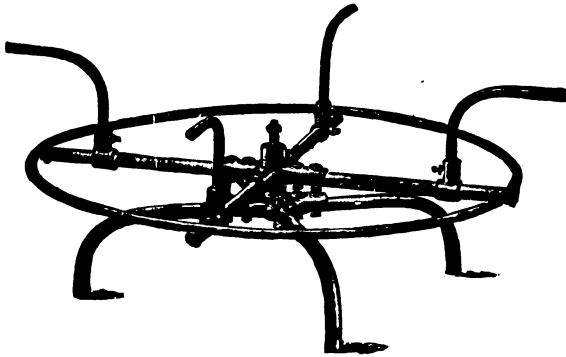
FIG. 111.— WIRE REEL.
