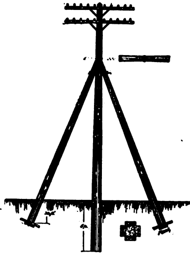
FIG. 104.— DOUBLE BRACE.
