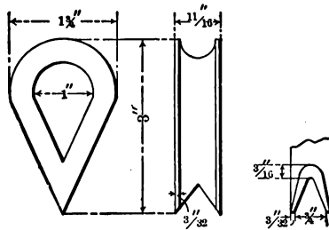
FIG. 74.— THIMBLE.
