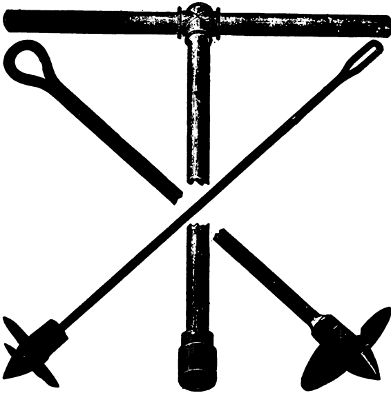
FIG. 95.—GUY ANCHOR.
