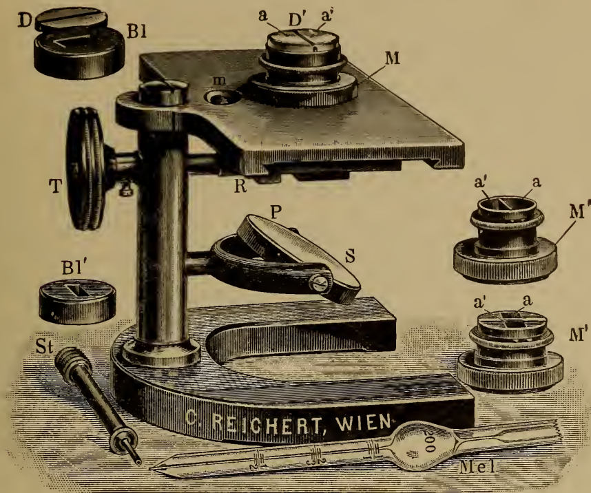
FIG. 9. Fleischl-Miescher hemometer.
