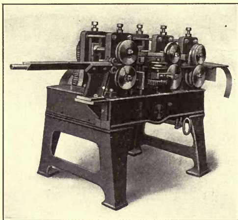
FIG. 123.— Pipe rolling machine.
