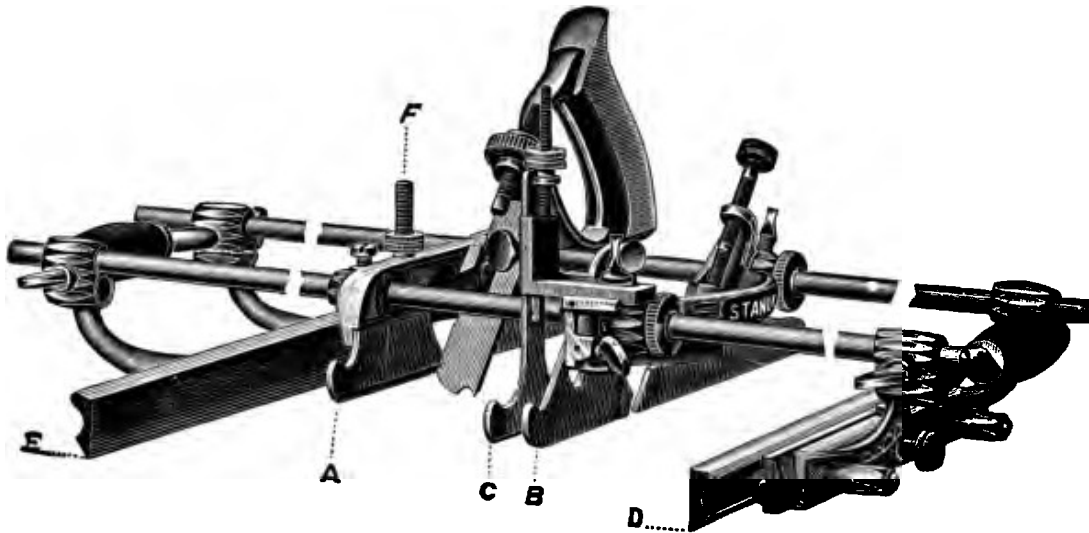
Fig. 117. Universal Plane.
