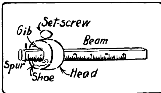
Fig. 211. Marking-Gage.
