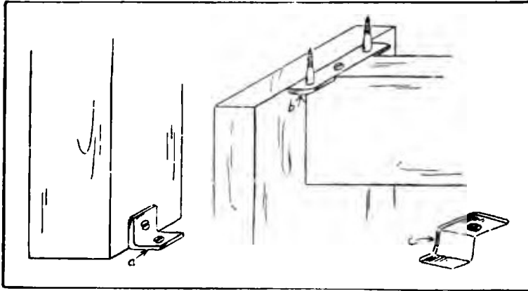
Fig. 232. a. Corner-iron. b. Straight plate. c. Panel-iron.
