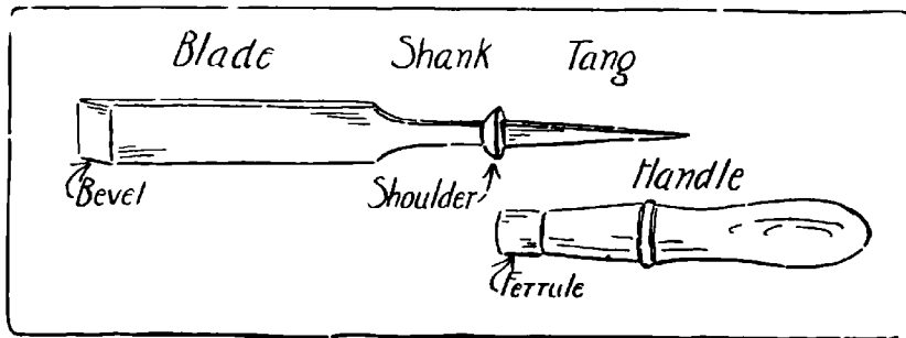
Fig. 65. Firmer-Chisel.
