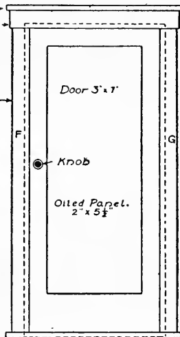
FIG 89 FRONT DOOR
