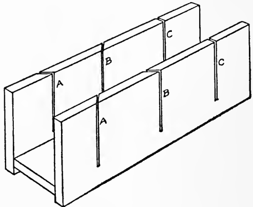
FIG. 12. — A Mitre-box.
